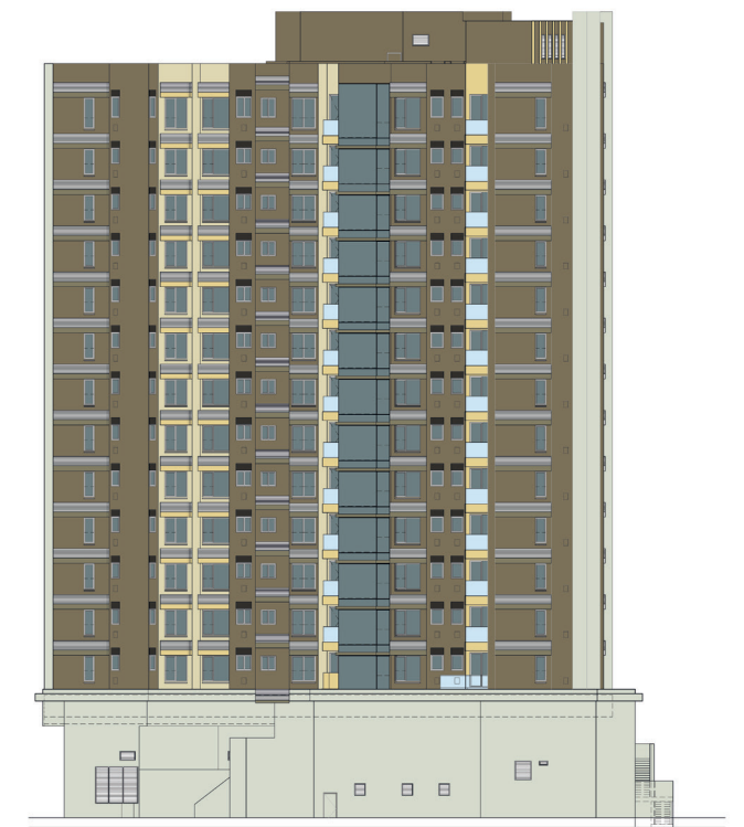
4 第1座北面立面 Tower 1 North Elevation
